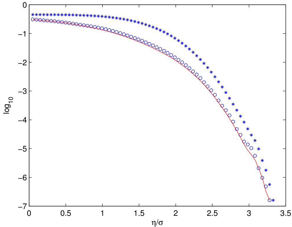
Duffing oscillator \zeta=2\% , \lambda=5
