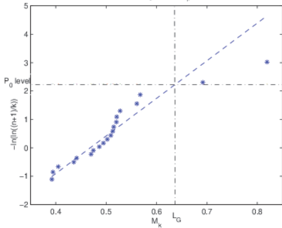
Gumbel plot H_s=14.7\text{m} , T_p=16.5\text{s}
