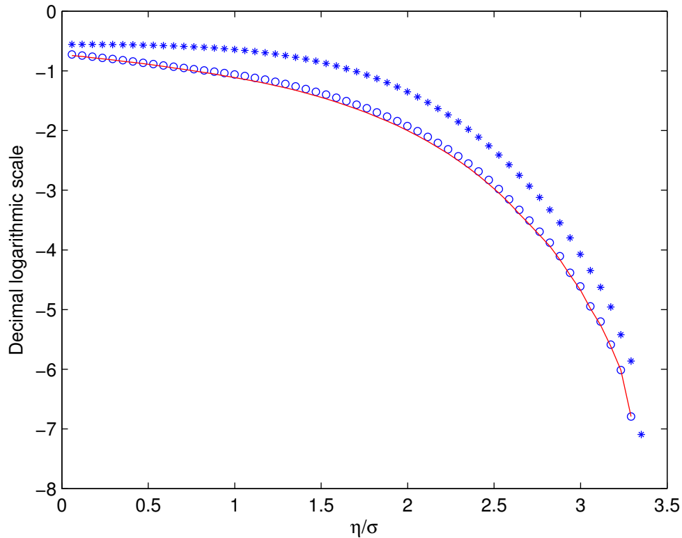
Duffing oscillator \zeta=2\% , \lambda=1
