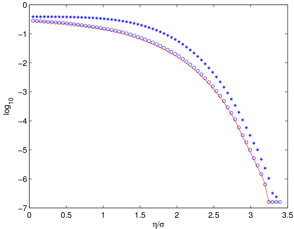
Duffing oscillator \zeta=4\% , \lambda=5
