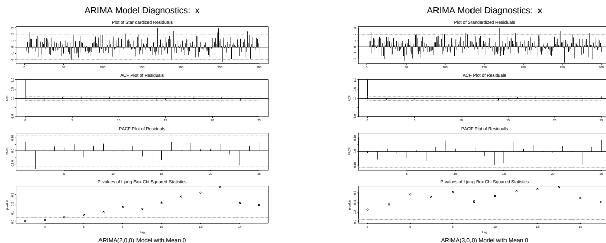
Figur 3: Modelldiagnoseringsplott for de tilpassede AR(2)- og AR(3)-modellene.
